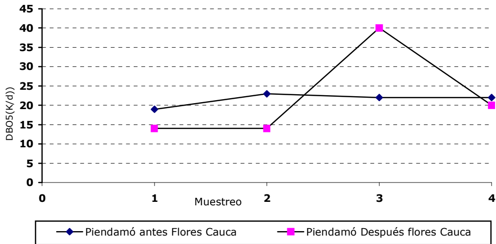
Gráfico 27. Carga contaminante para DBO 5 , Microcuenca de la Quebrada Los Vivos
