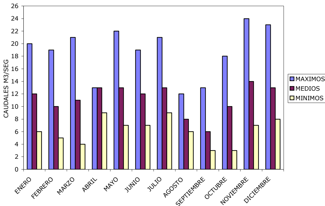
Gráfico 16. Caudales (Q) medios del río Piendamó. Estación Guaicondo, periodo 1983-1993
