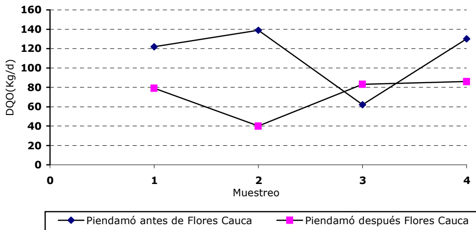
Gráfico 28. Cargas contaminantes para DQO Microcuenca de la Quebrada Los Vivos
