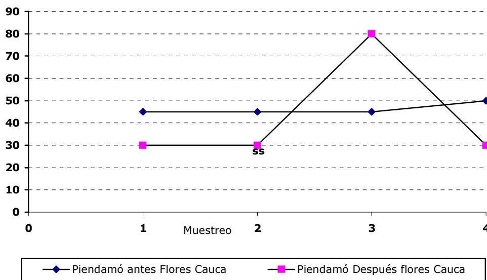
Gráfico 29. Cargas contaminantes para SST Microcuenca de la Quebrada Los Vivas
