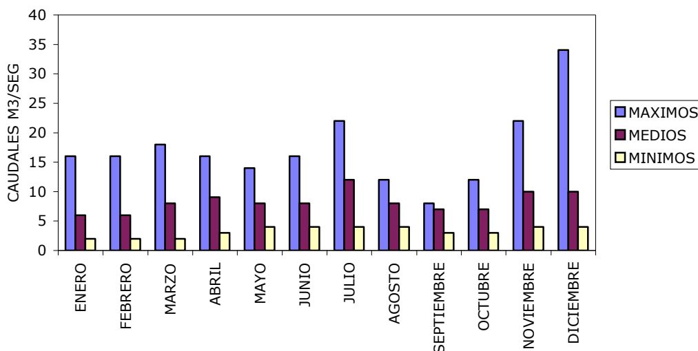
Gráfico 15. Caudales (Q) medios del río Piendamó. Estación Puente Carretera, periodo 1965-1990
