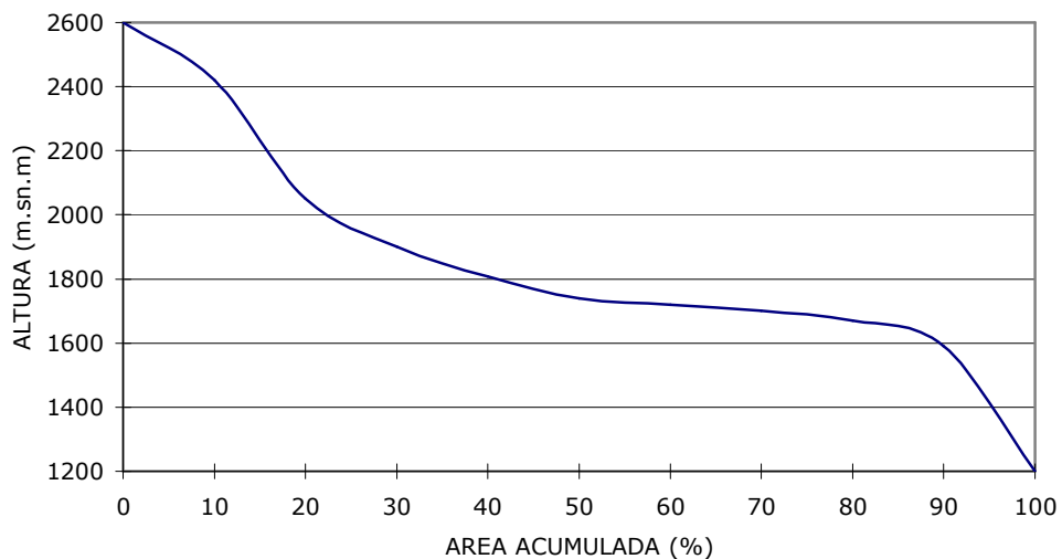
Gráfico 23. Curva hipsométrica Microcuenca del Río Pescador
